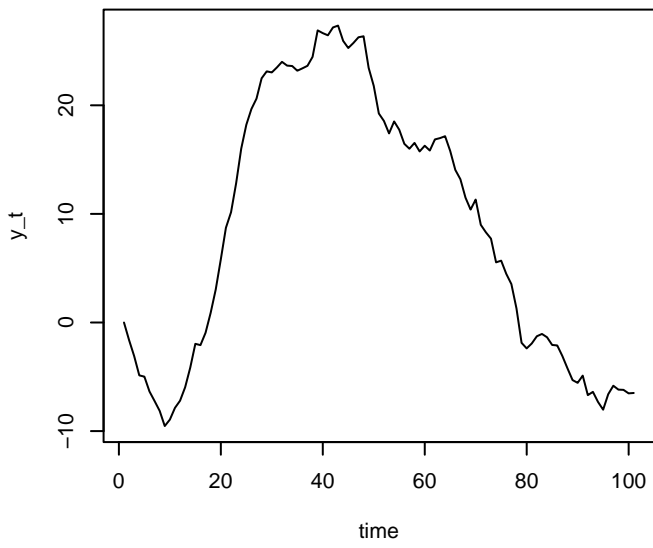
ARIMA(1,1,1)
